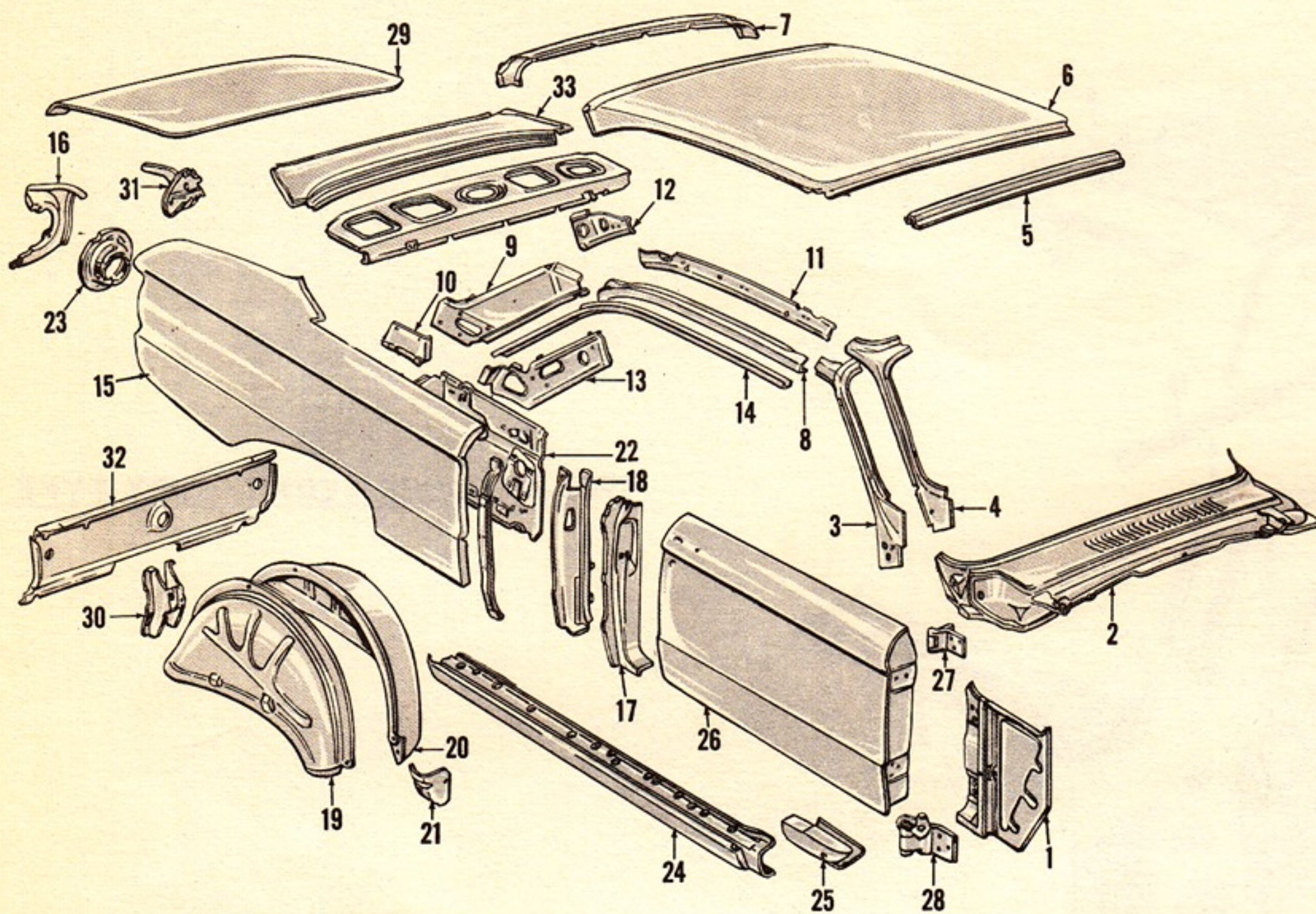
2- DOOR HARD TOP BODY PANELS
